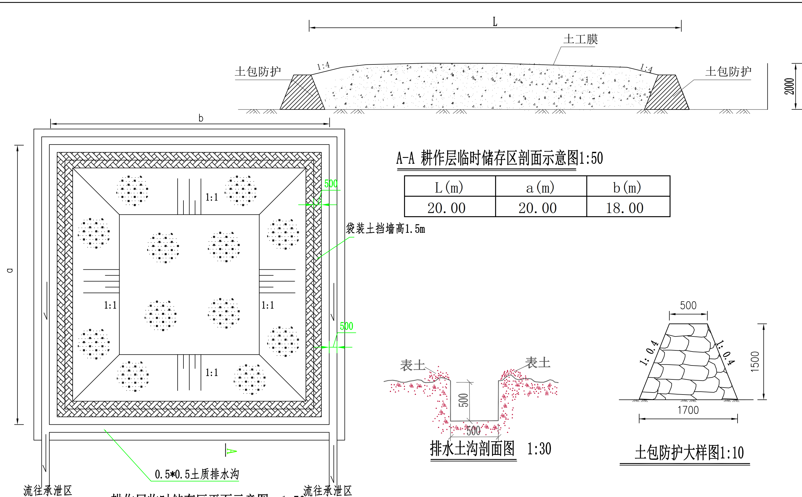
耕作层临时储存区平面示意图 1:50
