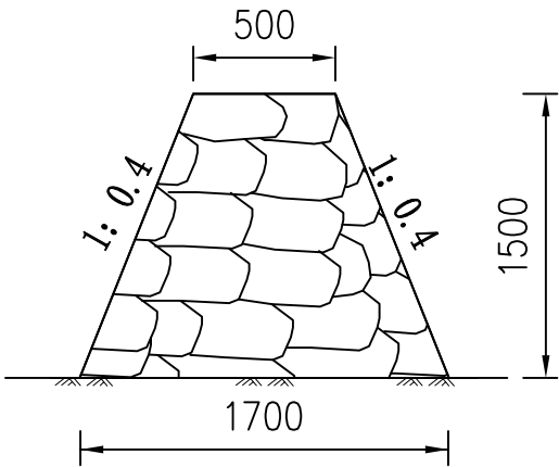
土包防护大样图1:10
