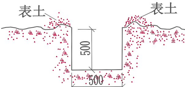
排水土沟剖面图 1:30
