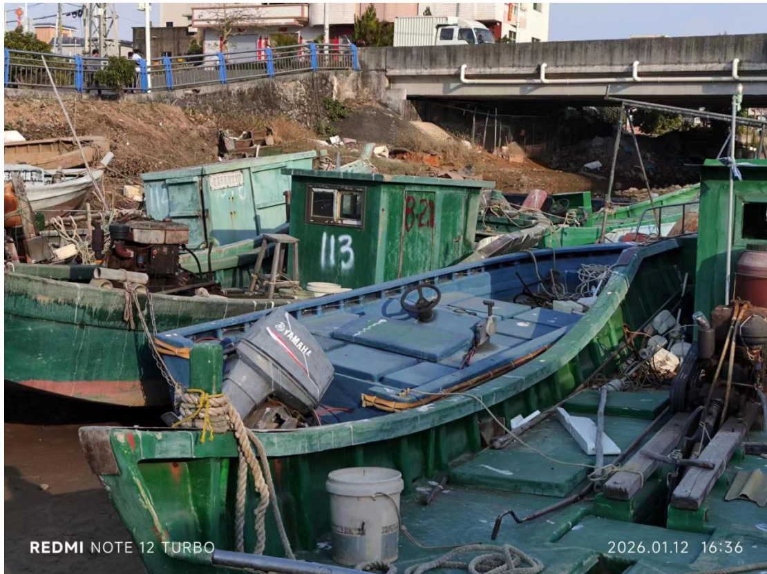
10. 编号: 112 (船长 7.2 米, 宽 1.8 米)
