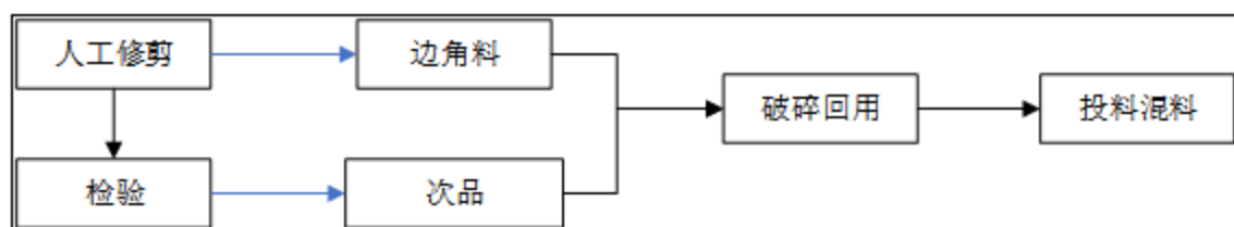
图 2-4 生产流程中破碎回用的工艺流程示意图
