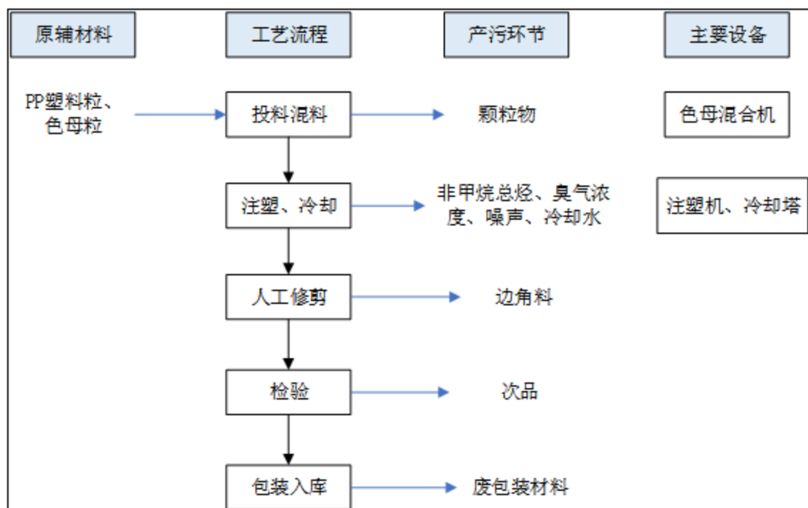
图 2-2 聚丙烯 (PP) 容器生产工艺流程及排污节点示意图
