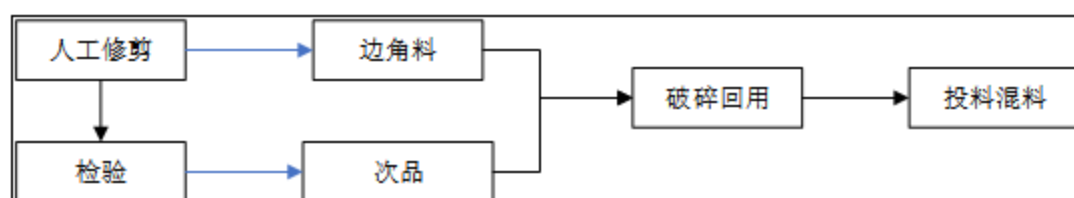
图 2-6 生产中破碎回用的工艺流程示意图
