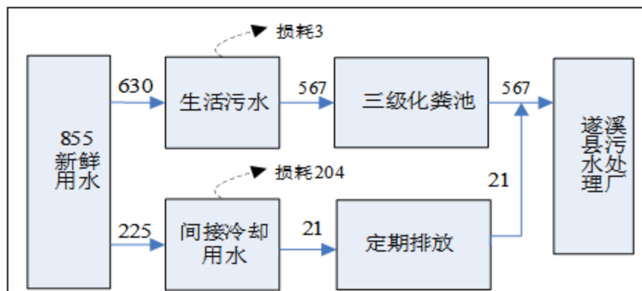
图 2-2 水平衡图 (单位: \text{m}^3/\text{a} )
