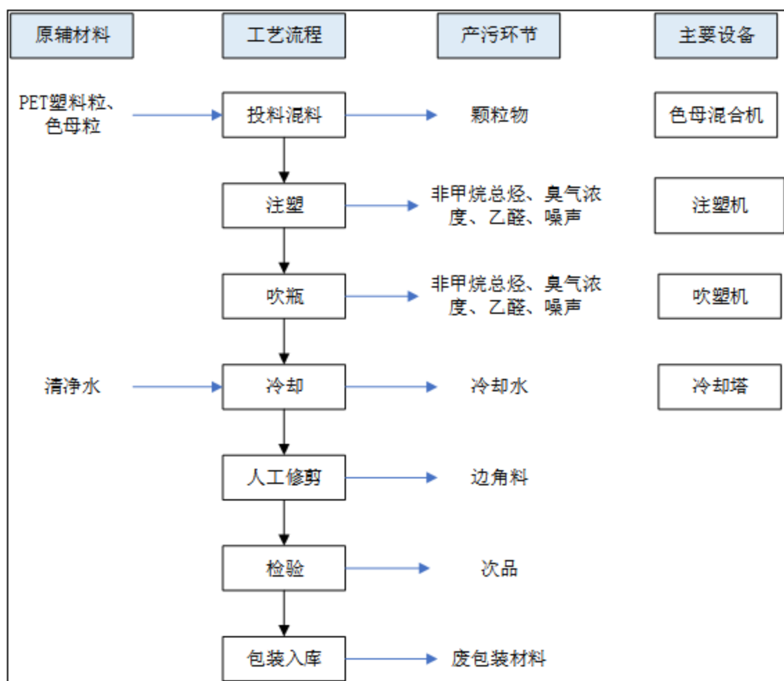
图 2-3 聚酯（PET）容器生产工艺流程及排污节点示意图
