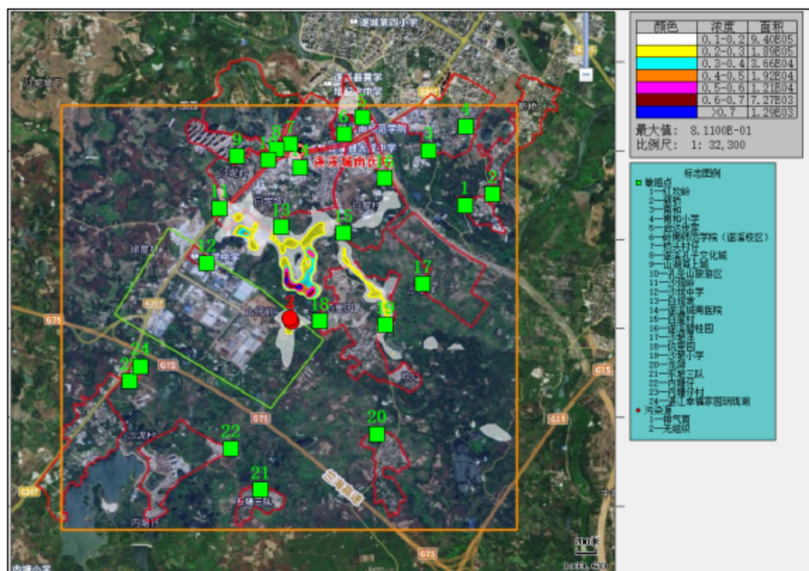
图 4.6 非甲烷总烃 1h 平均贡献浓度网格分布图 (单位: \text{mg}/\text{m}^3 )
