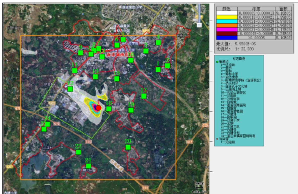
图 4.9 TSP 年平均贡献浓度网格分布图 (单位: \text{mg}/\text{m}^3 )
