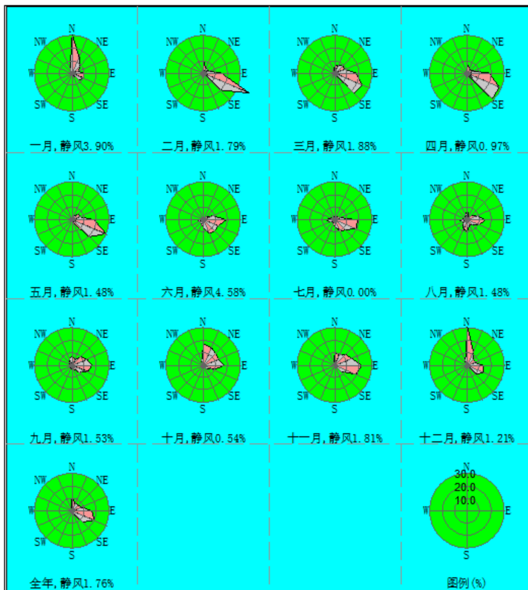
图 4.1 湛江 2023 年平均风频玫瑰图
