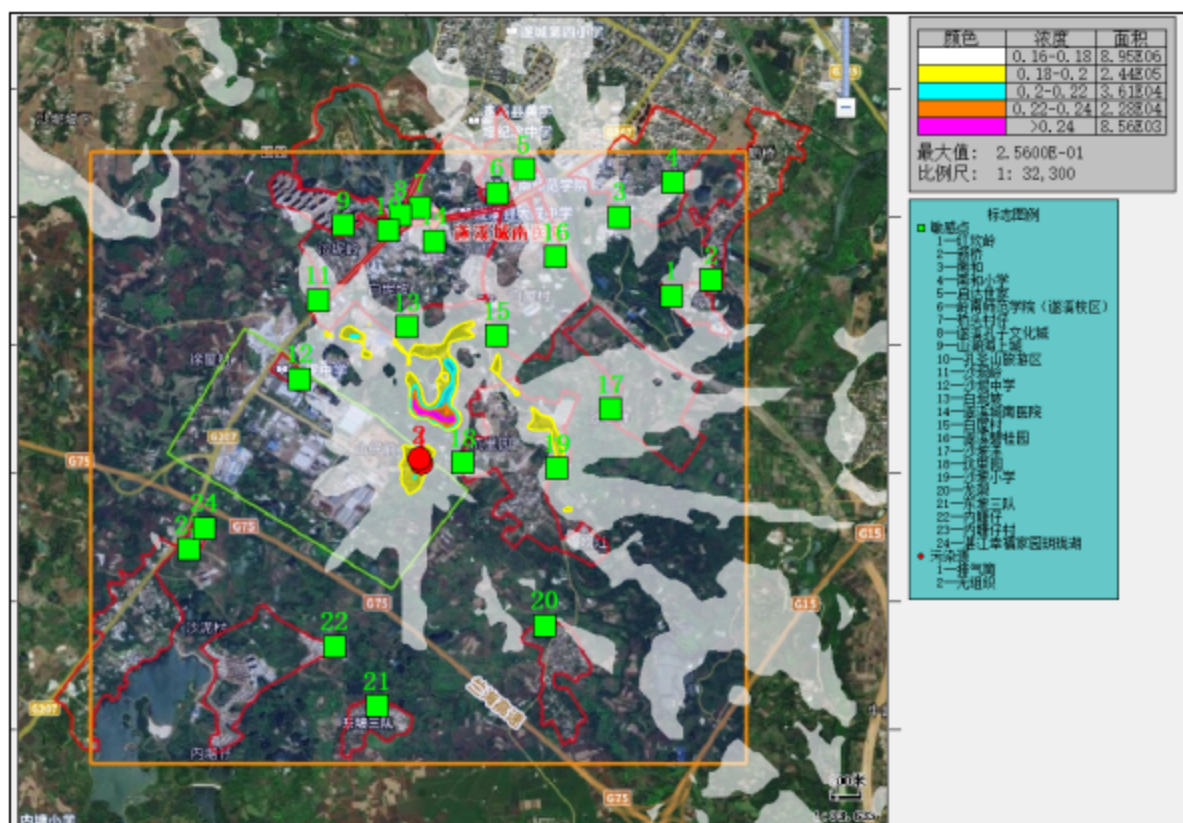
图 4.24 TVOC 8h 平均叠加浓度网格分布图(单位: mg/m 3 )
