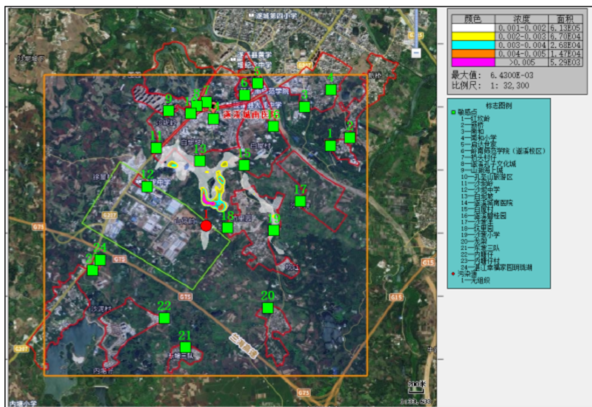
图 4.10 PM_{10} 1h 平均贡献浓度网格分布图(单位: mg/m^3 )
