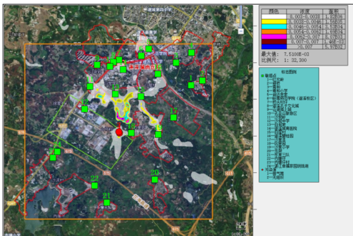
图 4.17 乙醛小时叠加浓度网格分布图(单位: \text{mg}/\text{m}^3 )
