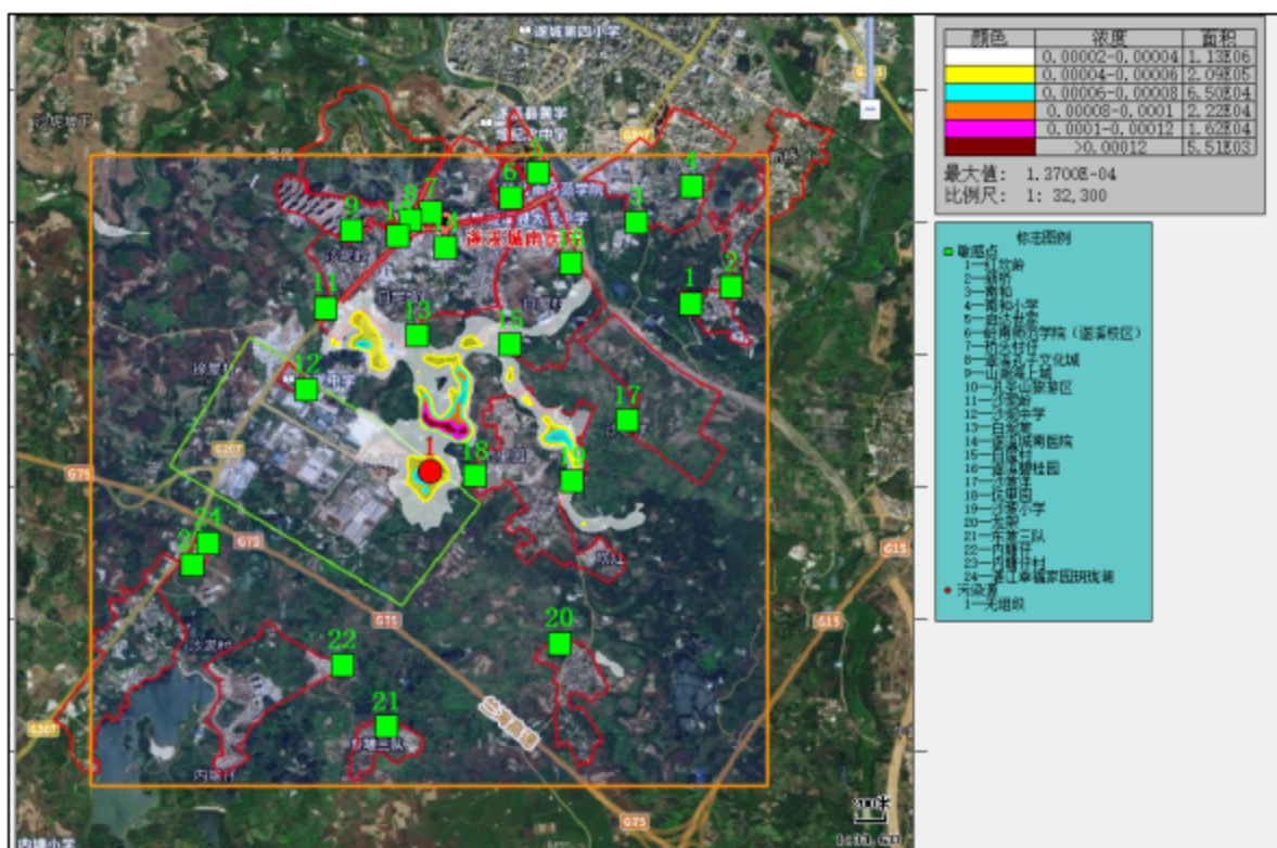
图 4.14 PM 2.5 日平均贡献浓度网格分布图(单位: mg/m 3 )
