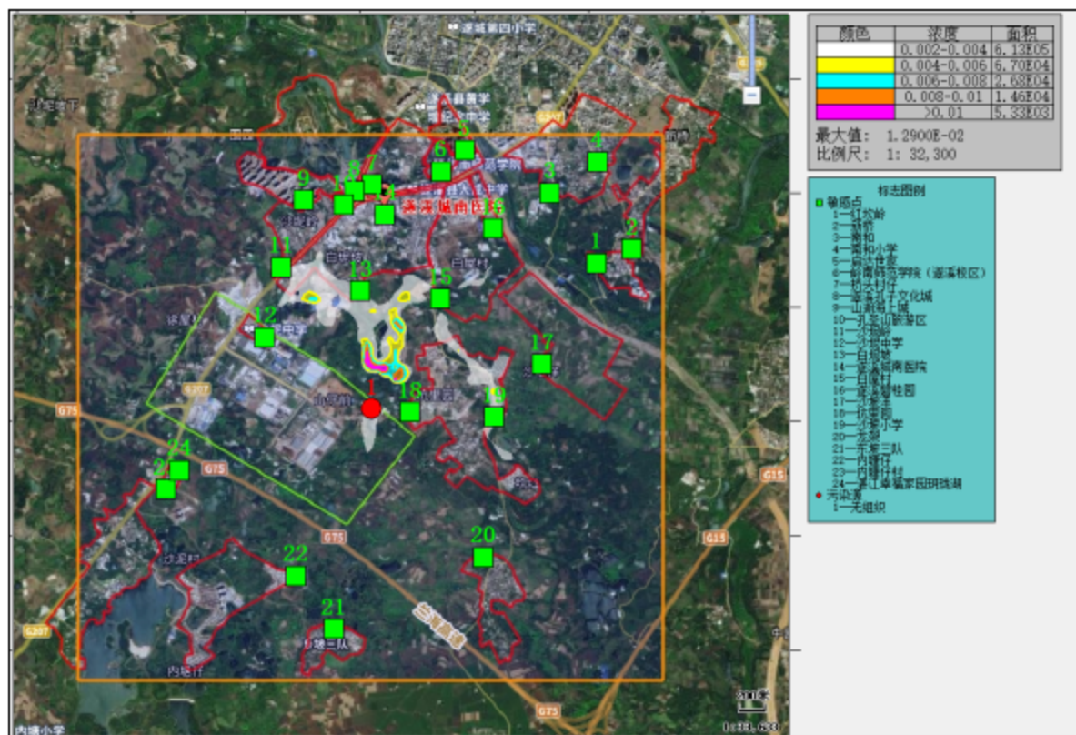
图 4.7 TSP 1h 平均贡献浓度网格分布图(单位: \text{mg}/\text{m}^3 )
