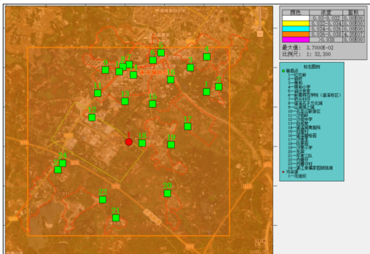
图 4.21 PM_{10} 年平均叠加浓度网格分布图(单位: mg/m^3 )
