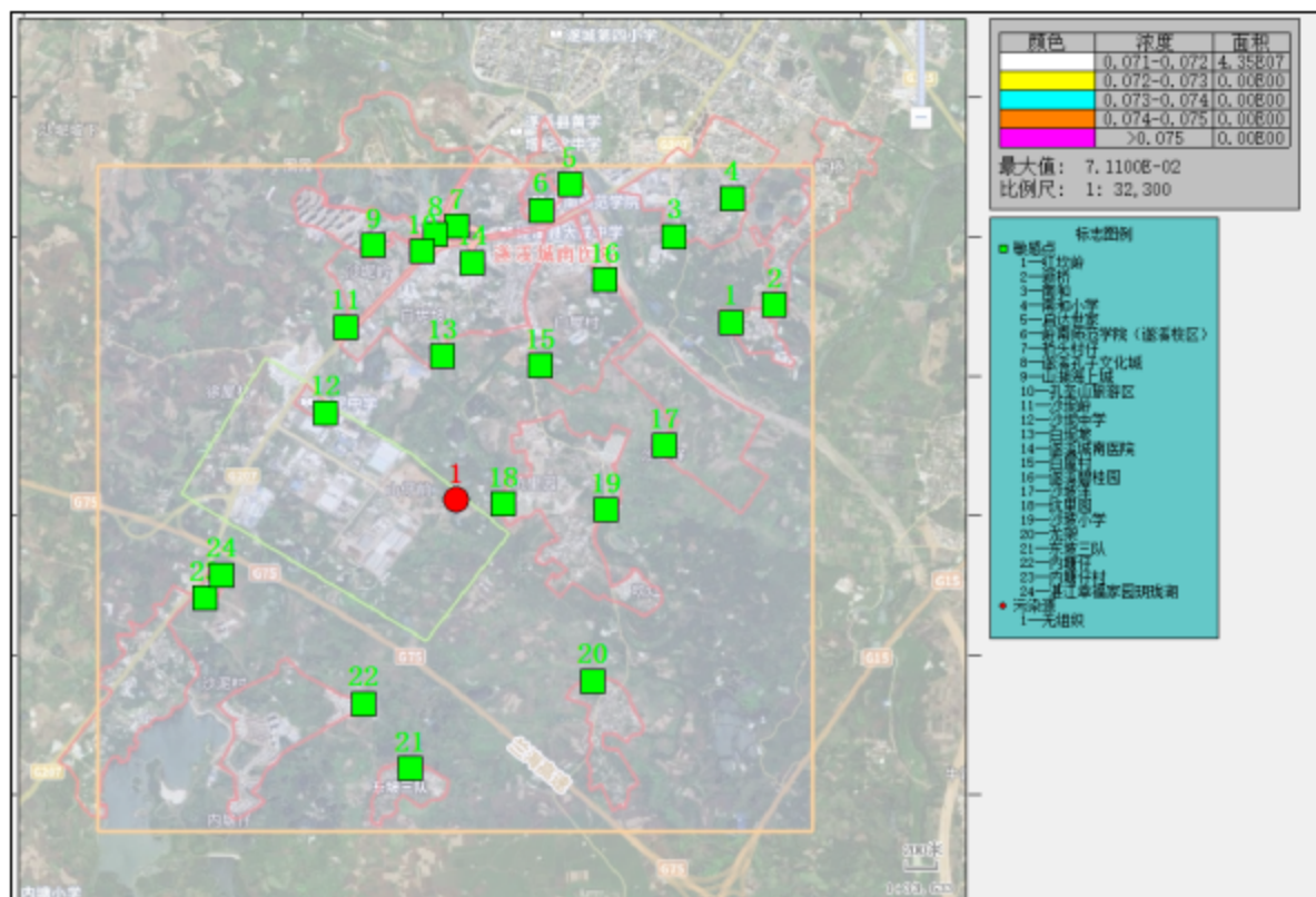
图 4.20 \text{PM}_{10} 第 95 百分位日平均叠加浓度网格分布图(单位: \text{mg}/\text{m}^3 )
