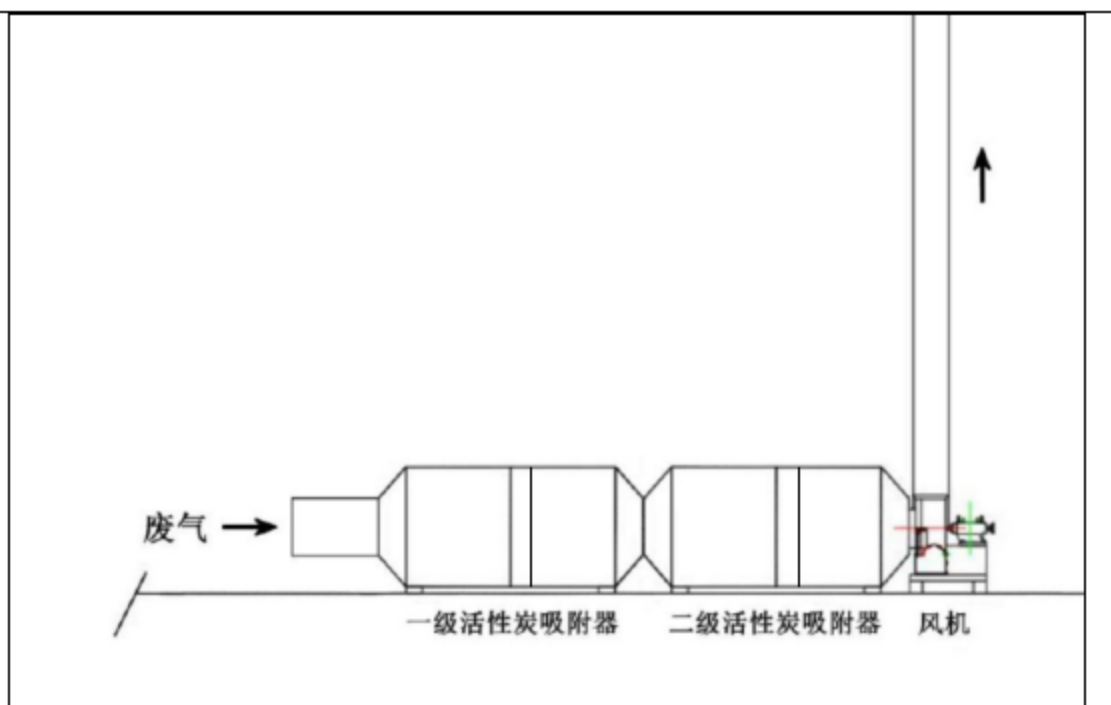
图 4-4 活性炭结构示意图
