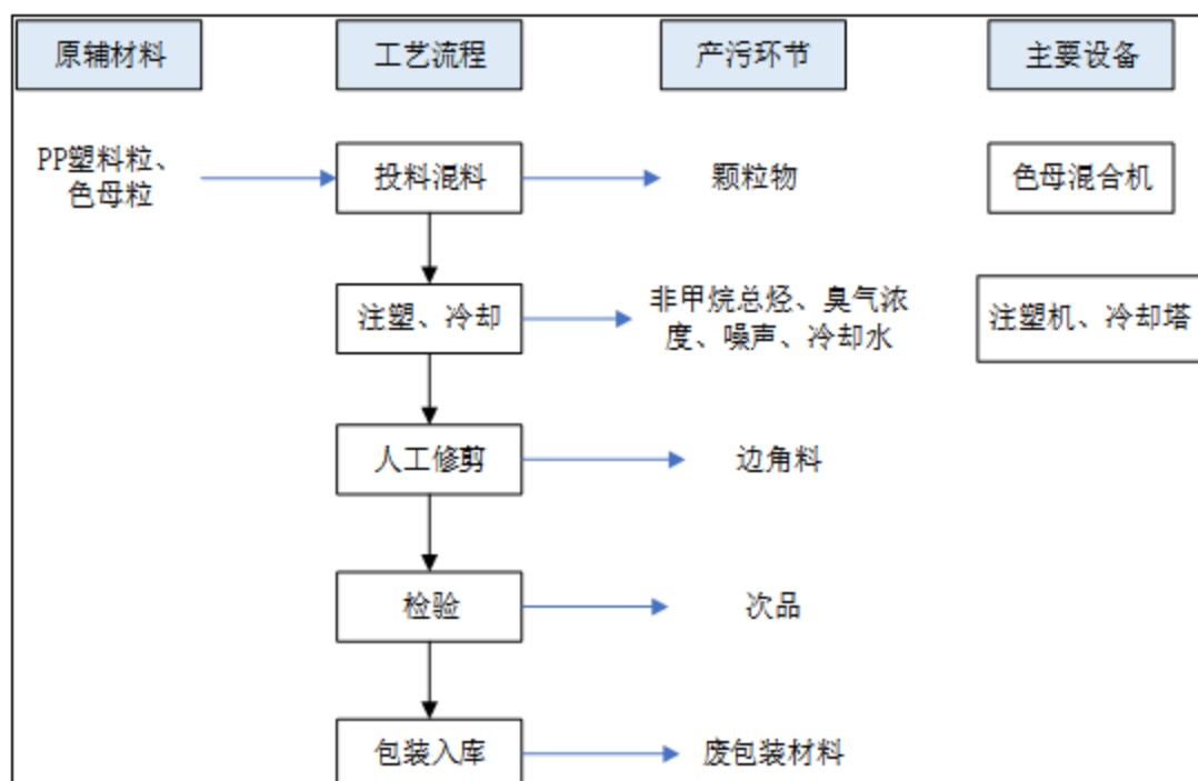
图 2-4 聚丙烯(PP)容器生产工艺流程及排污节点示意图
