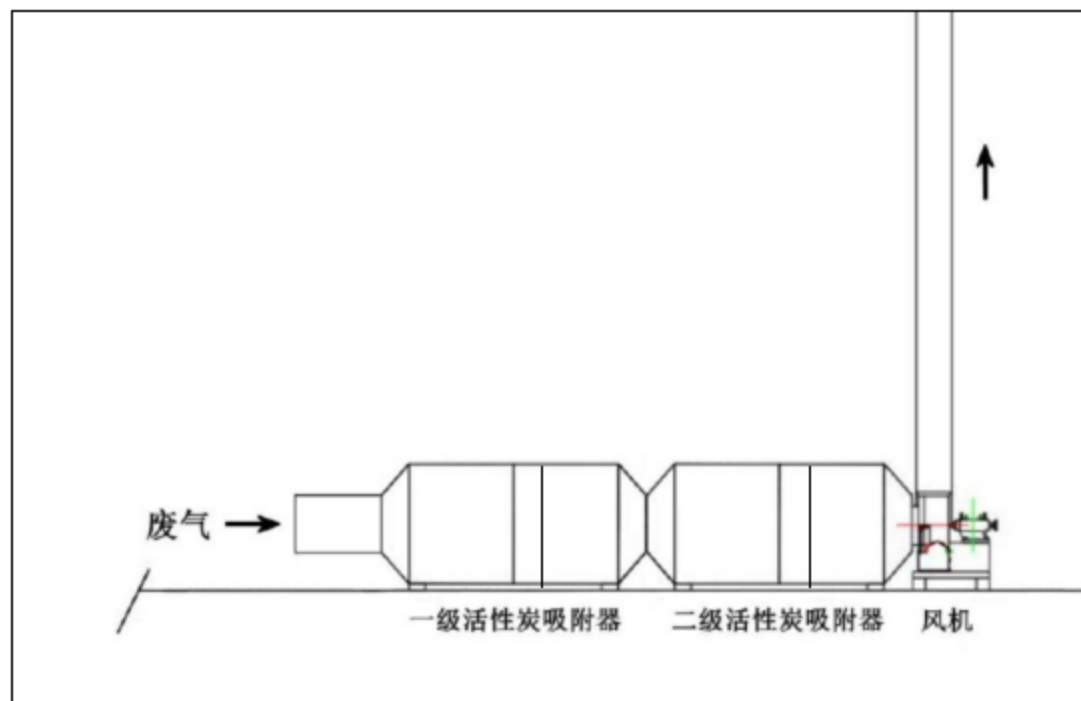
图5.2-1 活性炭吸附装置工作原理示意图
