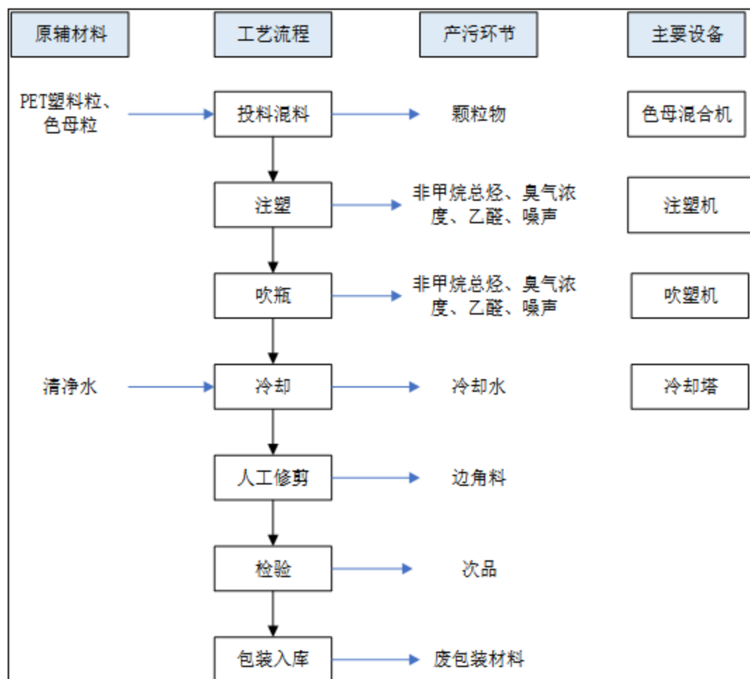
图 2-5 聚酯（PET）容器生产工艺流程及排污节点示意图
