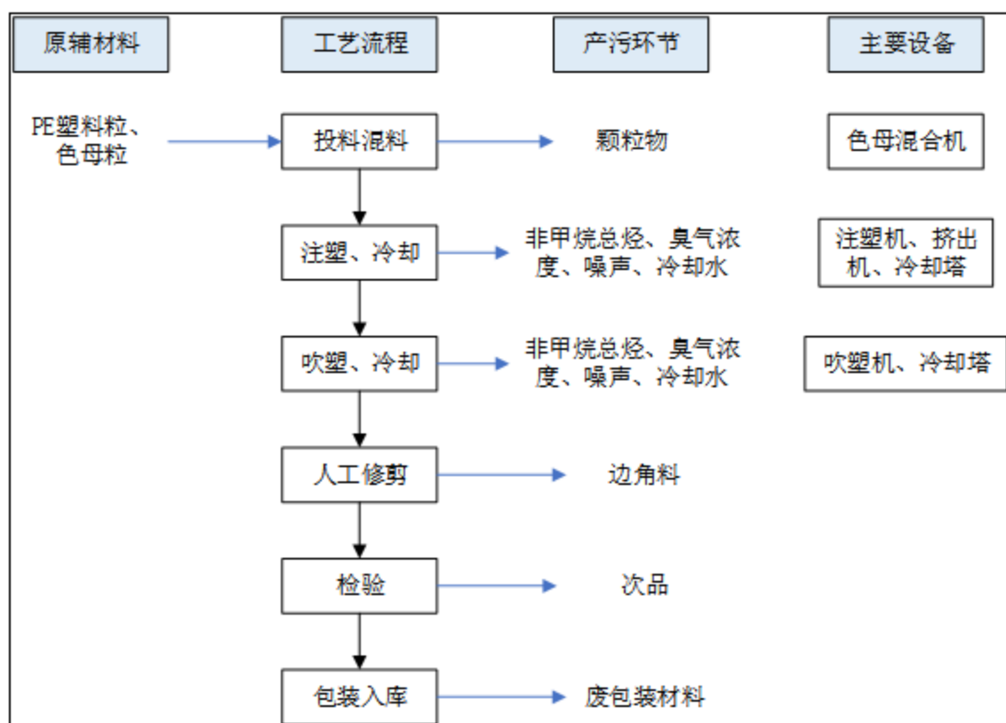
图 2-1 聚乙烯（PE）容器生产工艺流程及排污节点示意图
