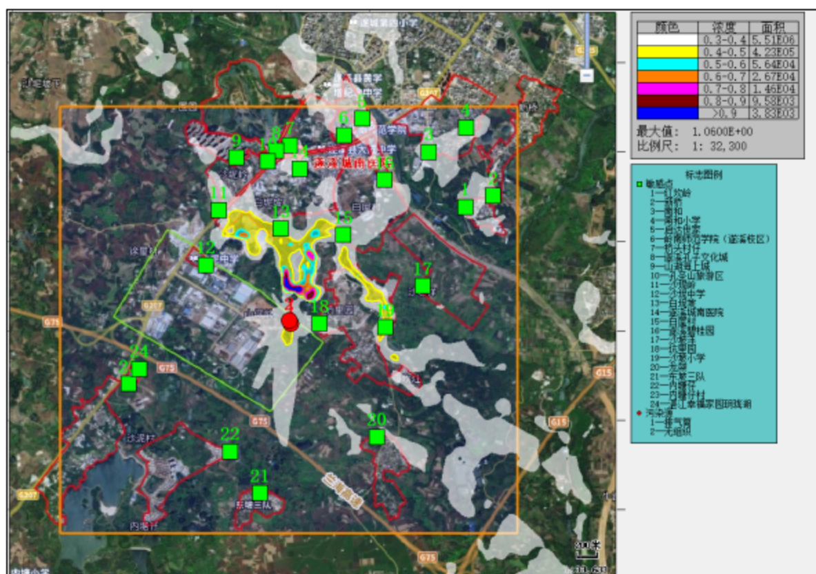
图 4.18 非甲烷总烃 1h 平均叠加浓度网格分布图(单位: \text{mg}/\text{m}^3 )
