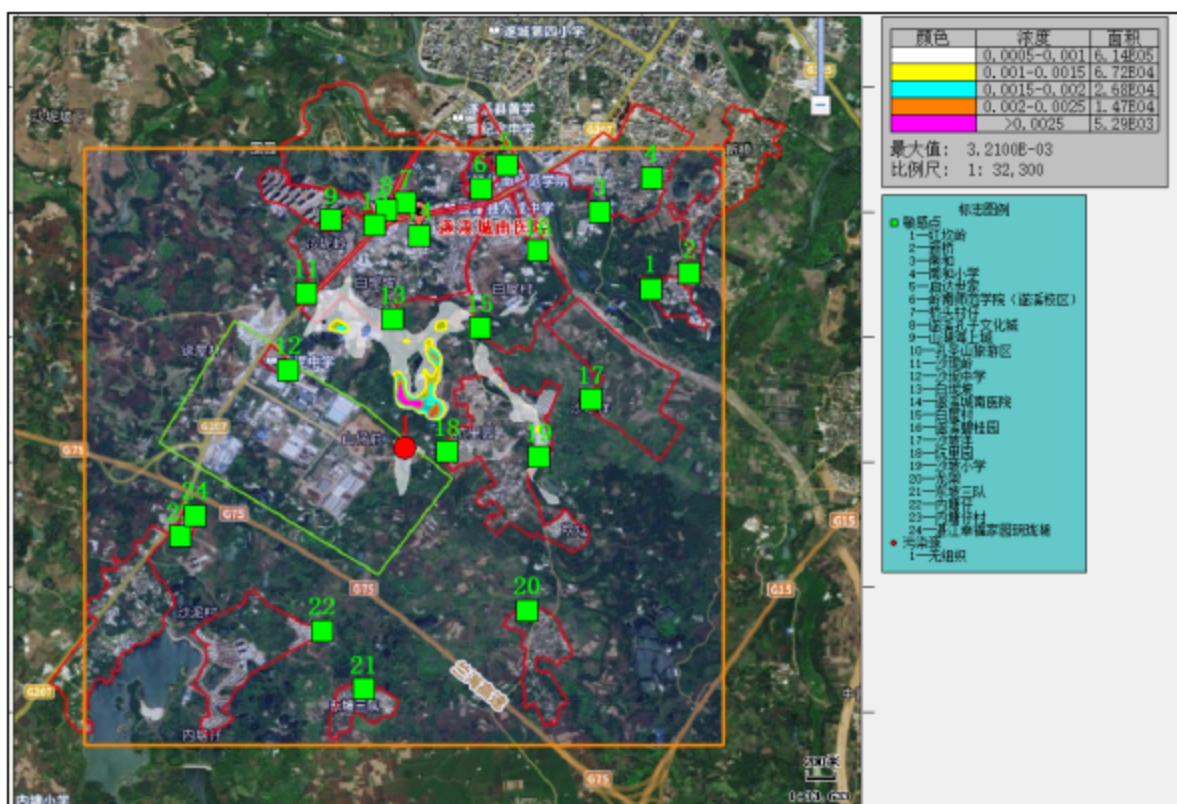
图 4.13 PM 2.5 1h 平均贡献浓度网格分布图(单位: mg/m 3 )
