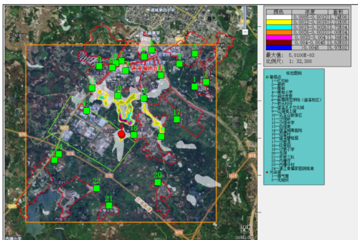
图 4.5 乙醛 1h 平均贡献浓度网格分布图 (单位: \text{mg}/\text{m}^3 )
