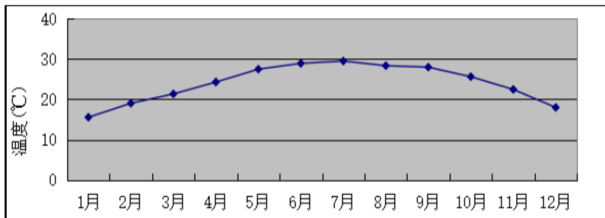
图 4.2 湛江 2023 年年均气温的月变化曲线图
