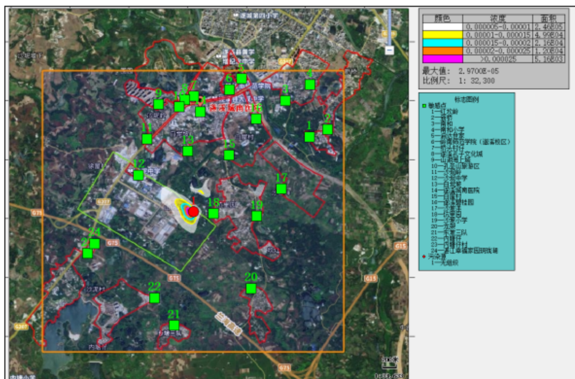
图 4.12 PM_{10} 年平均贡献浓度网格分布图 (单位: mg/m^3 )
