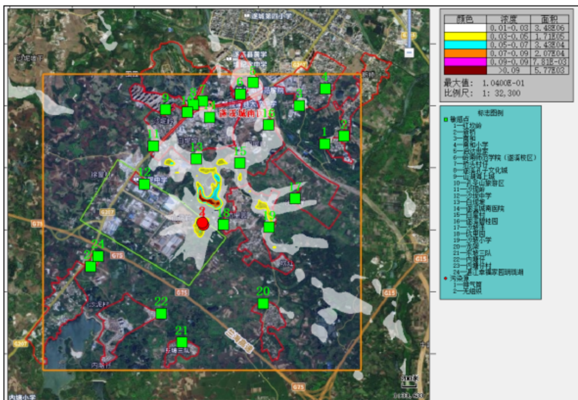
图 4.16 TVOCs 8h 平均贡献浓度网格分布图 (单位: mg/m^3 )
