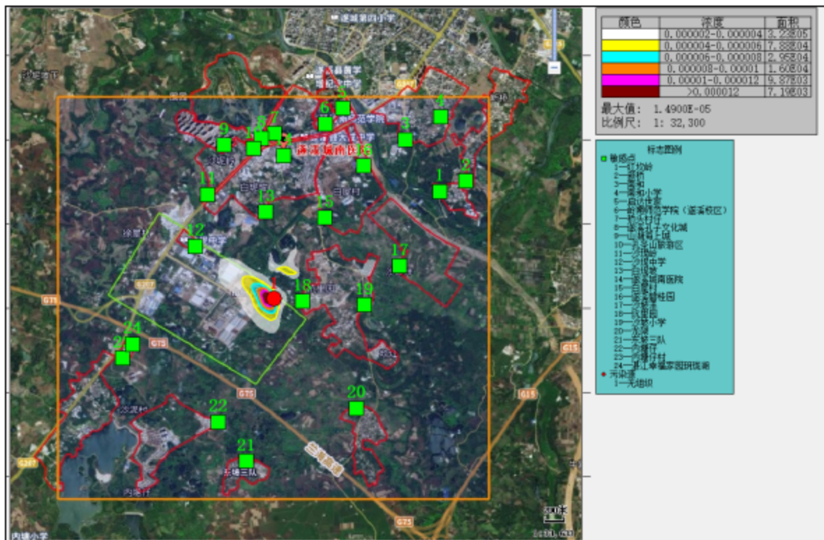
图 4.15 PM_{2.5} 年平均贡献浓度网格分布图 (单位: mg/m^3 )
