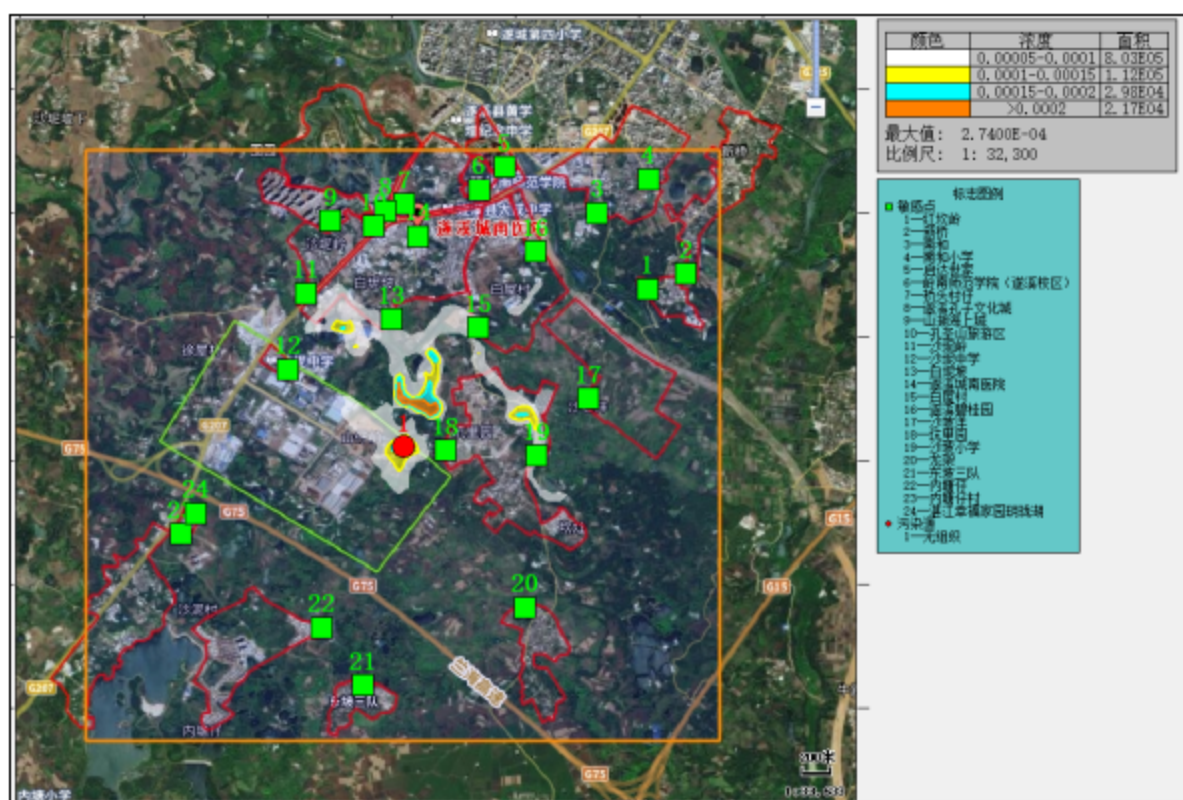
图 4.11 PM_{10} 日平均贡献浓度网格分布图(单位: mg/m^3 )
