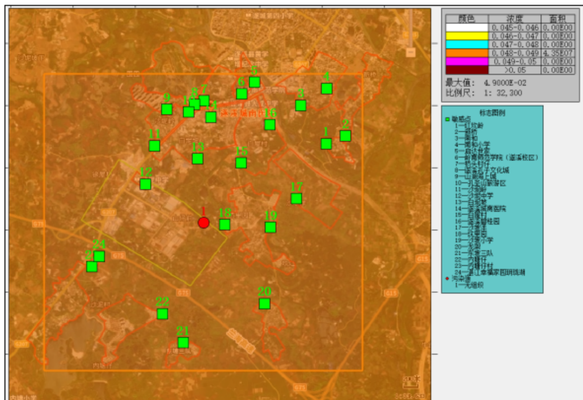
图 4.22 PM_{2.5} 第 90 百分位日平均叠加浓度网格分布图(单位: mg/m^3 )
