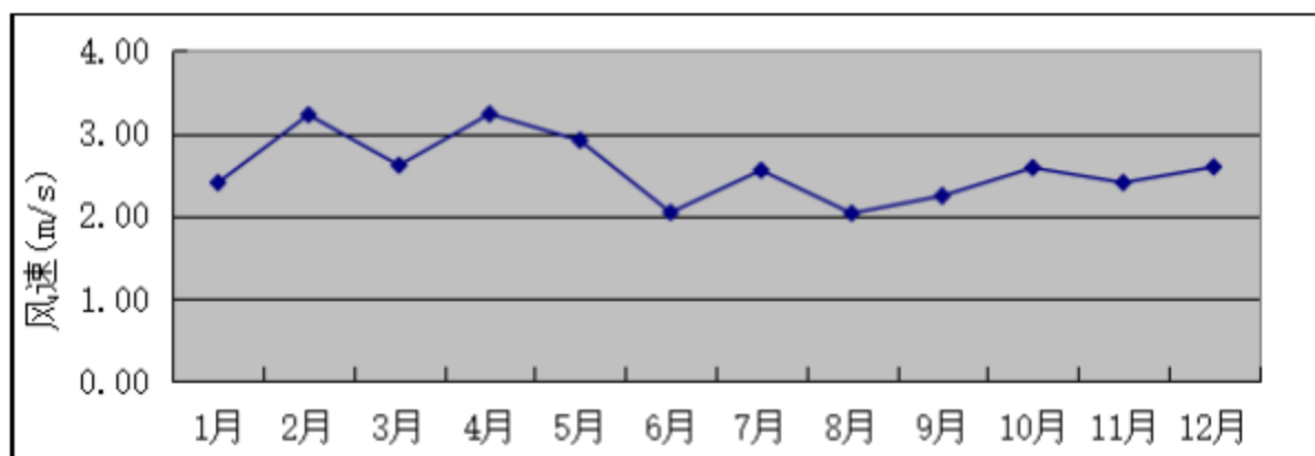
图 4.3 湛江 2023 年年均风速的月变化曲线图
