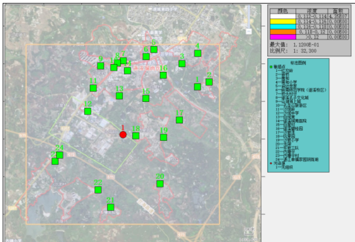
图 4.19 TSP 叠加最大浓度网格分布图(单位: \text{mg}/\text{m}^3 )
