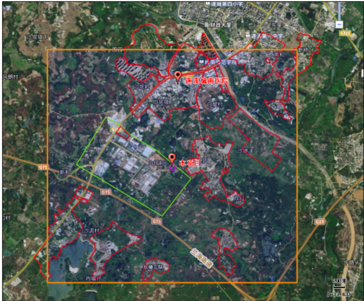
图 1.4-3 大气环境评价范围图
