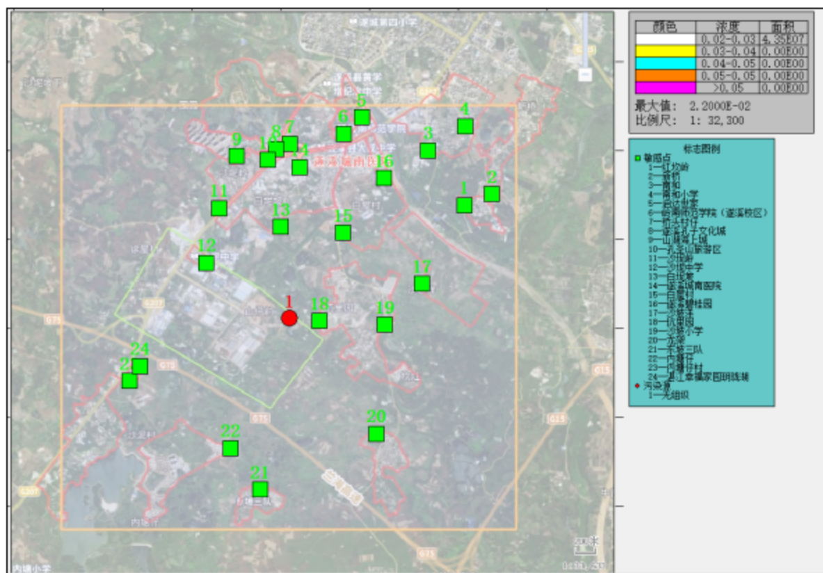
图 4.23 PM 2.5 年平均叠加浓度网格分布图(单位: mg/m 3 )
