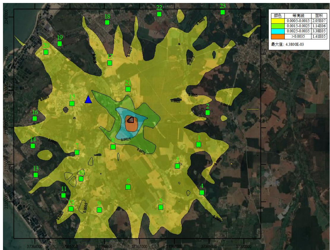
图 5.2.1-25 非正常工况下 H_2S 小时浓度预测值分布图
