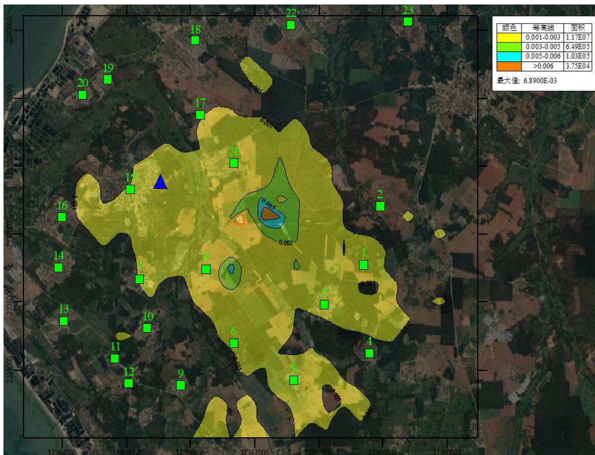
图 5.2.1-15 NO 2 小时浓度贡献值分布图
