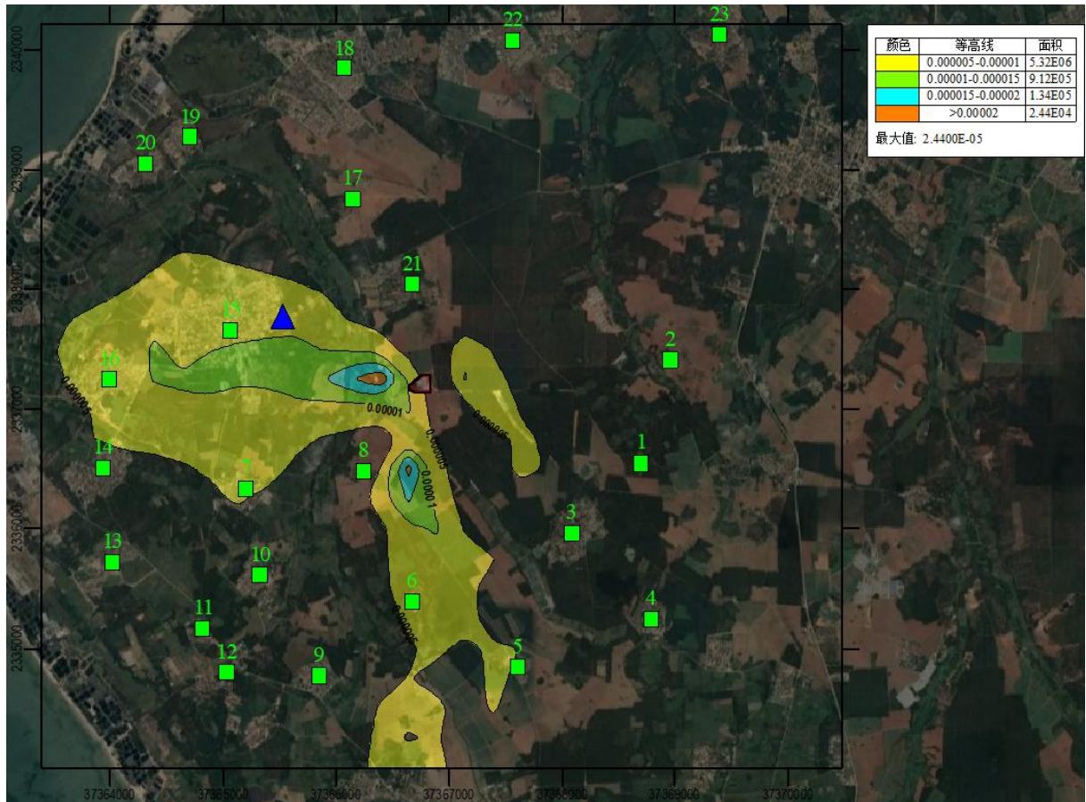
图 5.2.1-21 PM 2.5 年均浓度贡献值分布图
