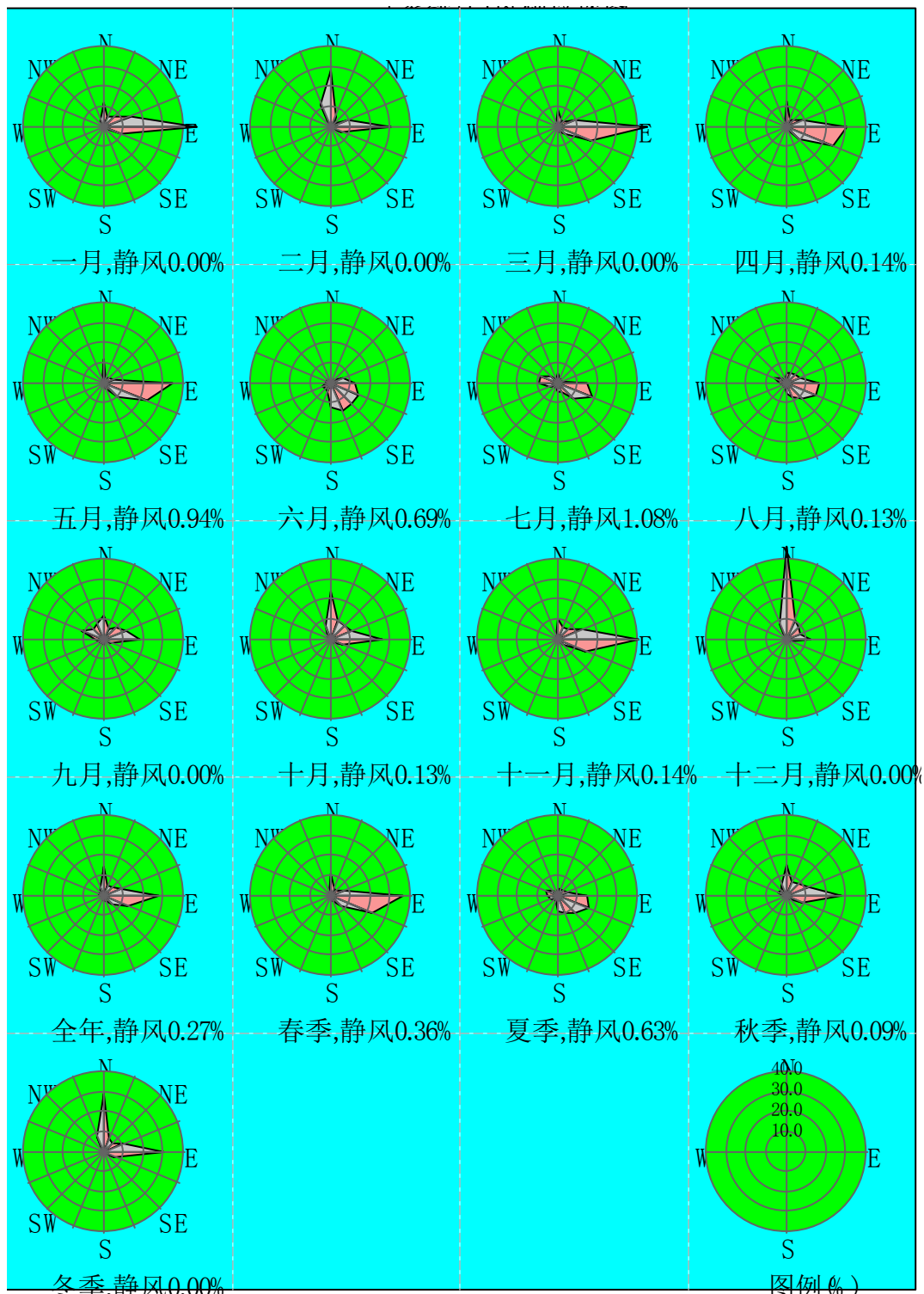
图 5.2.1-6 湛江市 2022 年地面风频玫瑰图
