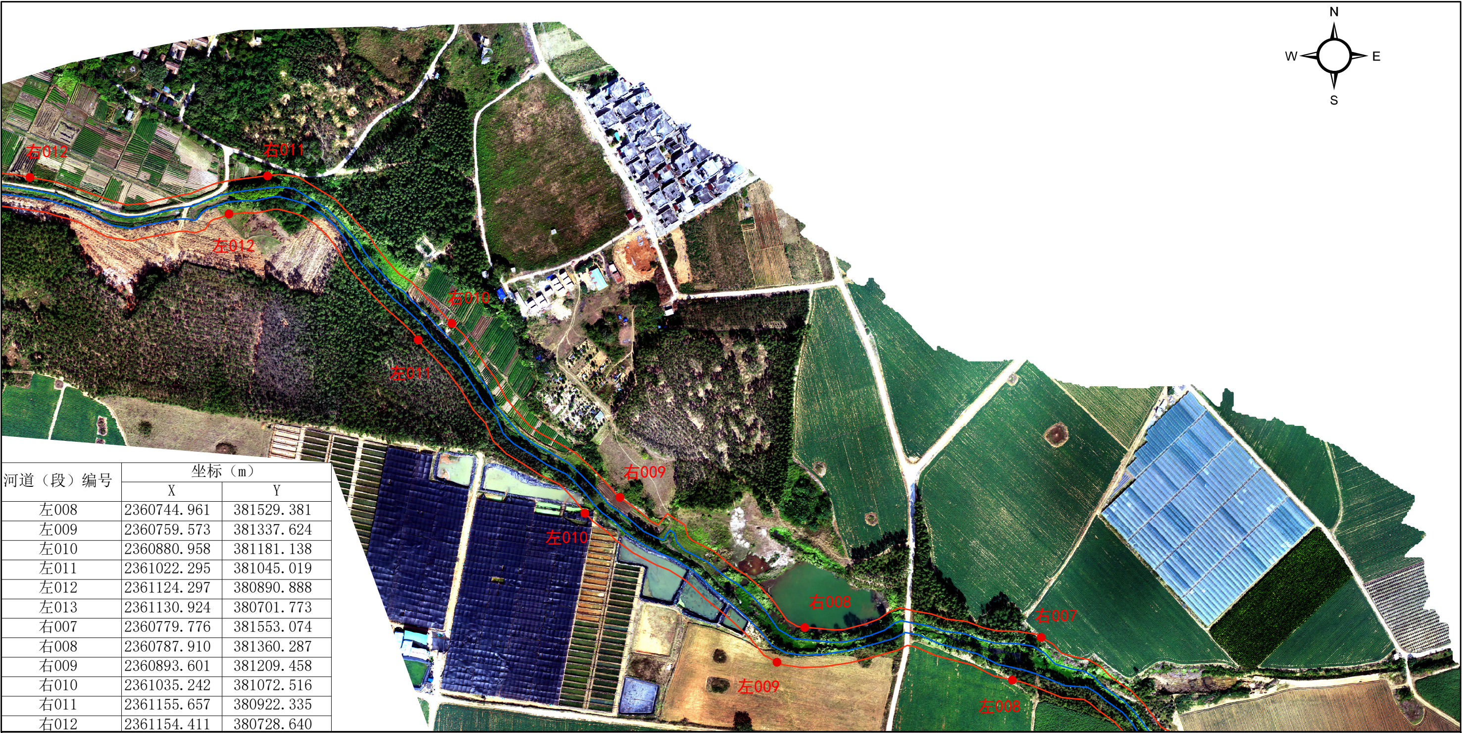
遂溪县那略沟管理范围划定成果图（3/4）
