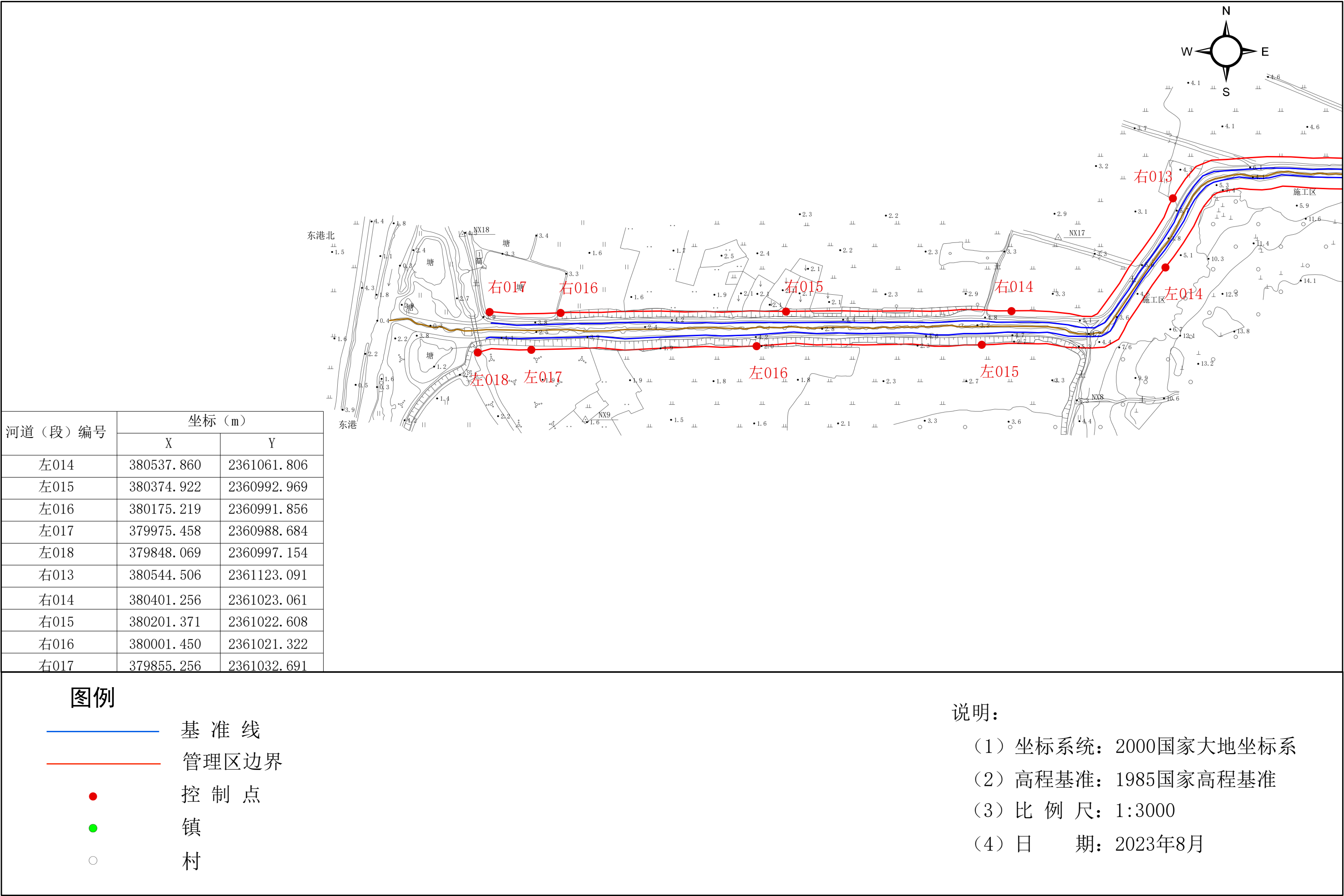
遂溪县那略沟管理范围划定成果图（4/4）
